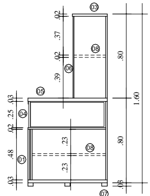
VISTA PAINEL LATERAL SEM ESCALA
