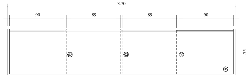
PLANTA BAIXA - PARTE INFERIOR SEM ESCALA
