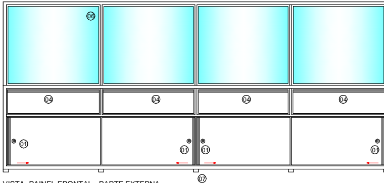
VISTA PAINEL FRONTAL - PARTE EXTERNA SEM ESCALA
